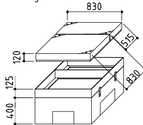
Ausführung II - Bkl. B auspflasterbar
