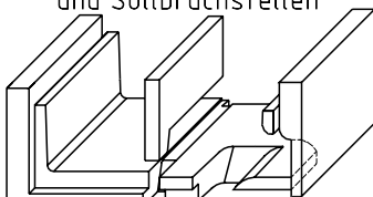
Sonderausführung mit Bodenaussparungen und Sollbruchstellen
